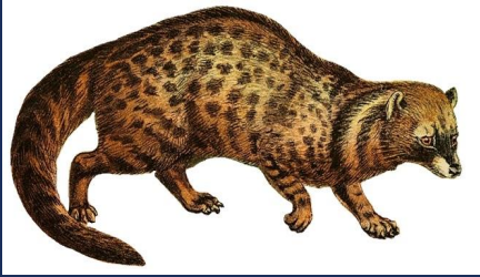
Civets 265
